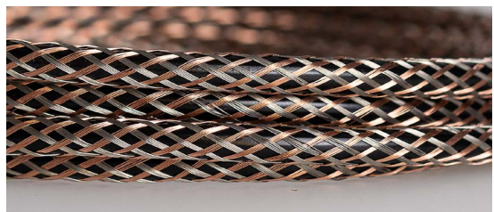
C60
